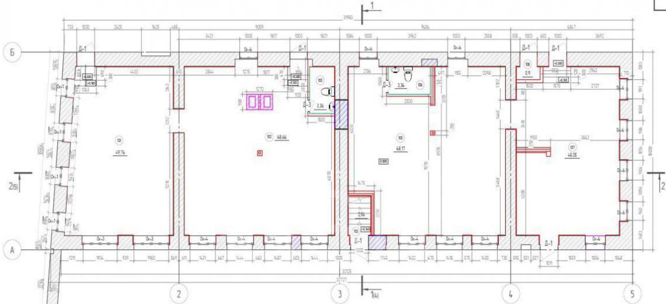
Экспликация помещений
