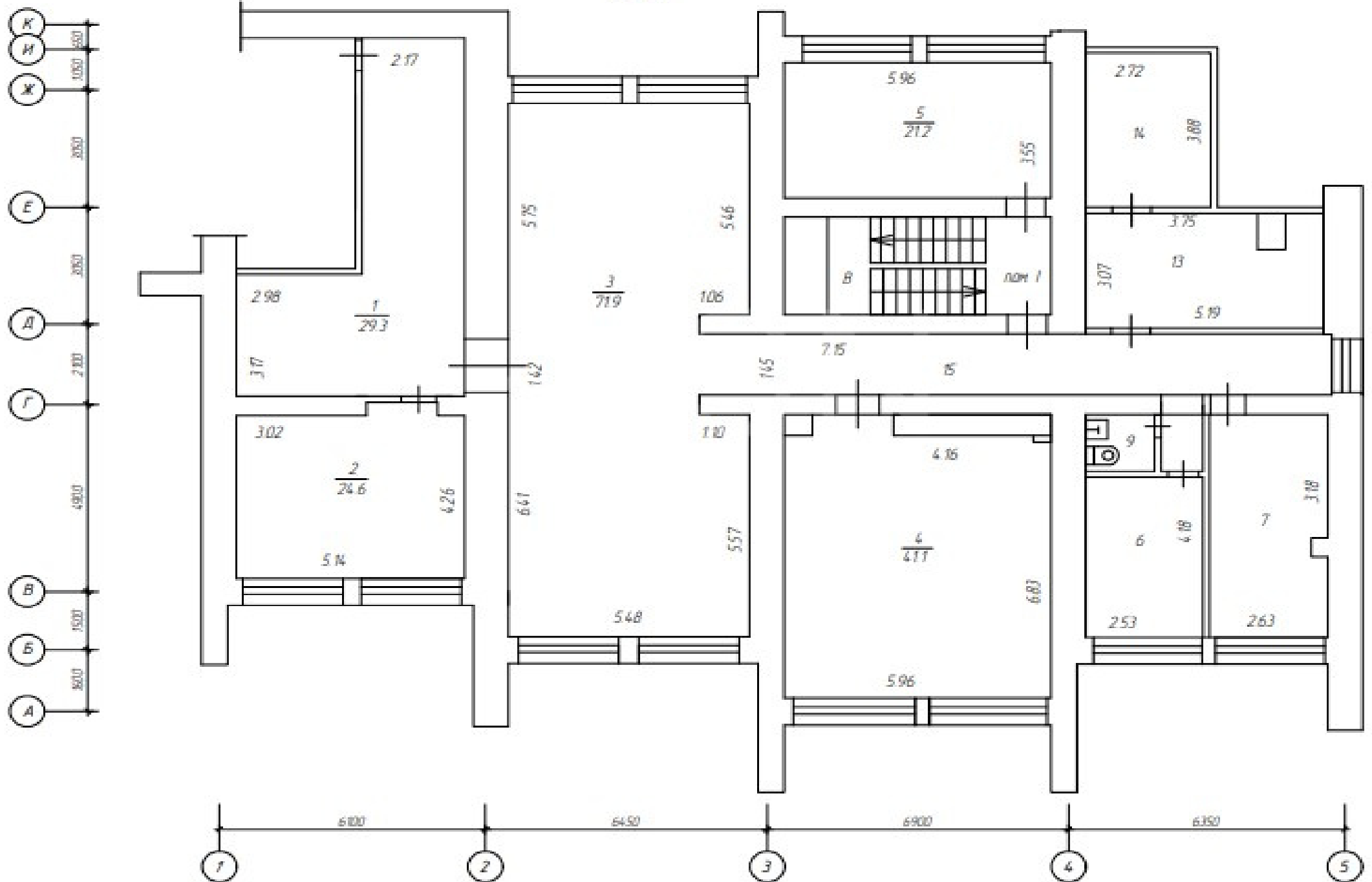
План помещения №1 с исходной конфигурацией помещения до переустройства и (или) перепланировки 2-й этаж М 1:100
