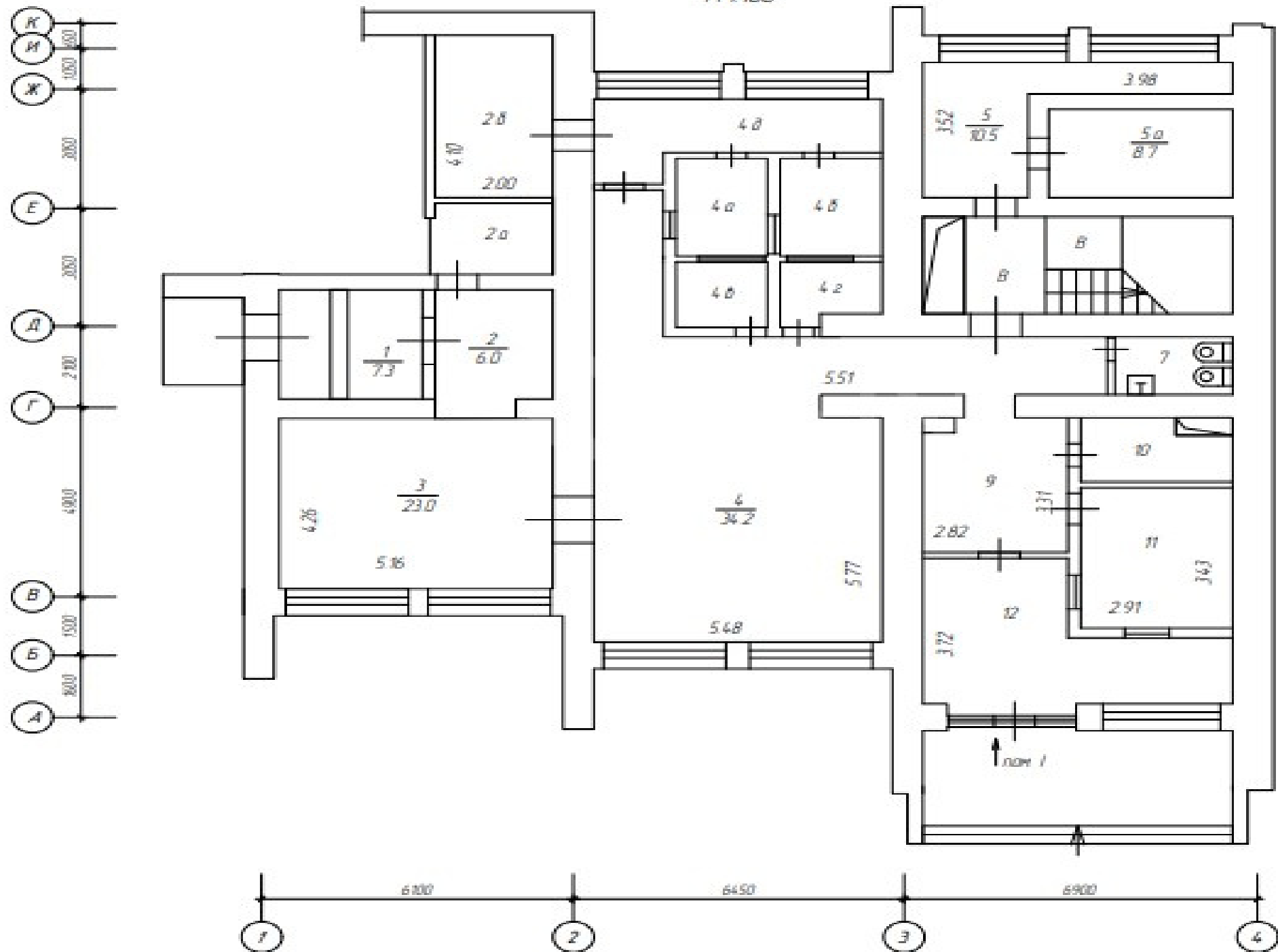
План помещения №9 с исходной конфигурацией помещения до переустройства и (или) перепланировки 1-й этаж М 1:100
