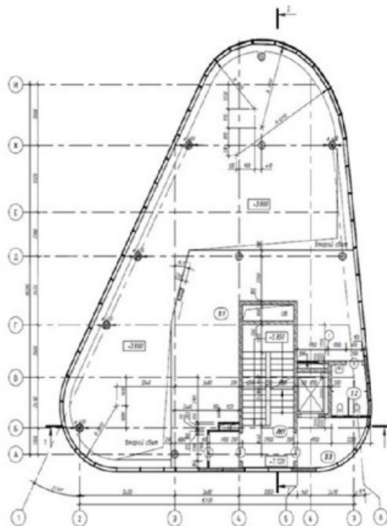
План антресольного этажа на отм. 7.800
