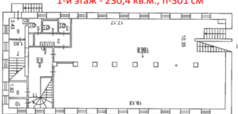
1-й этаж - 230,4 кв.м., h-301 см
