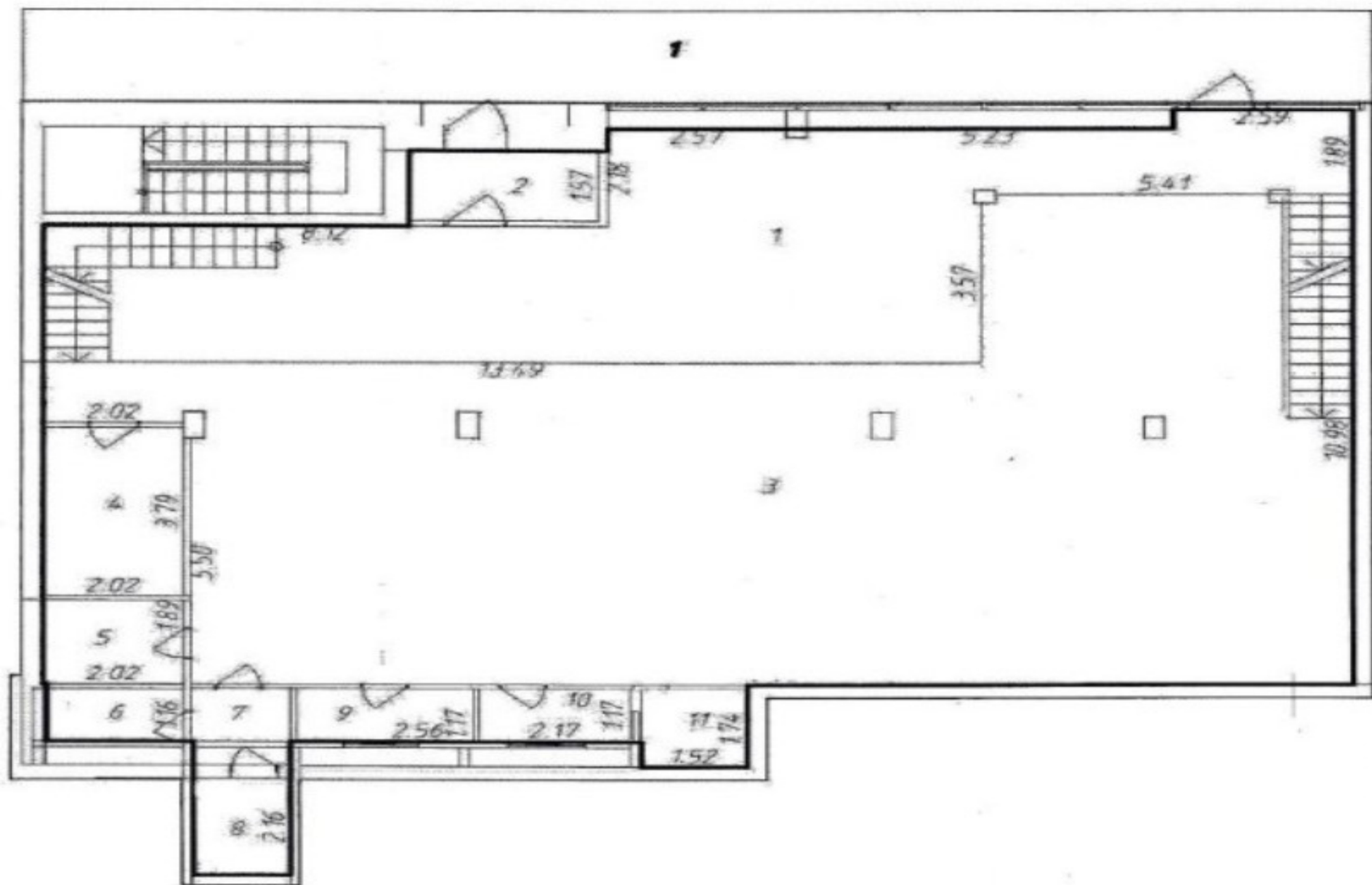
План цоколя этажа
