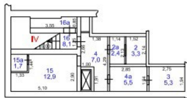
Подвальный Этаж
