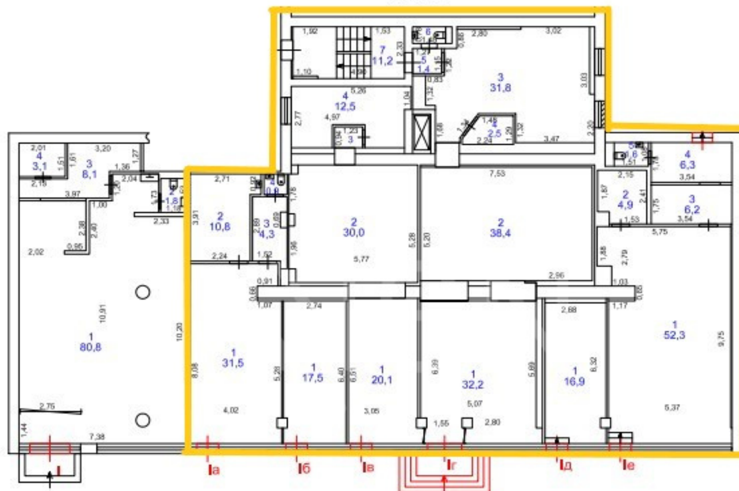
Подвальный Этаж
